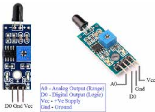
Fig. 4. Fire sensor
